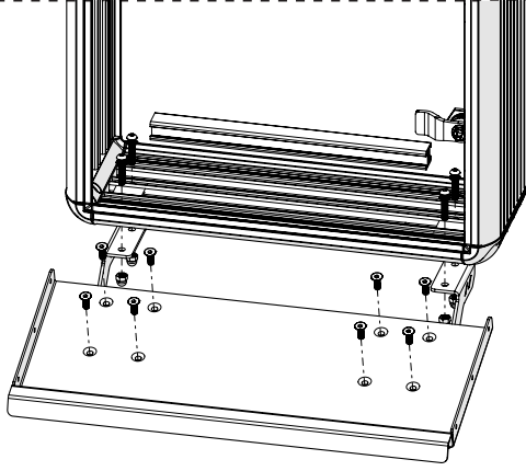
Mounting View Montaj Görünümü
