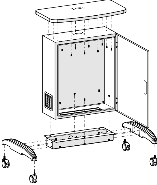
Mounting View Montaj Görünümü
