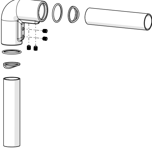
Mounting View Montaj Görünümü
