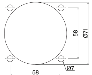
Panel mounting dimensions Pano montaj ölçüleri
