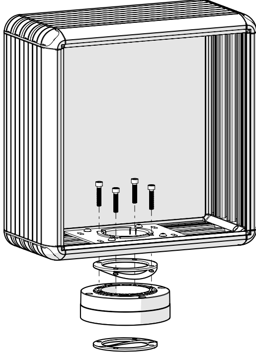
Mounting View Montaj Görünümü
