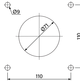
Ground mounting dimensions Zemin montaj ölçüleri
