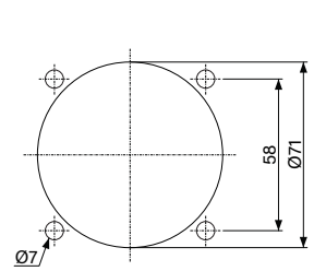
Panel mounting dimensions Pano montaj ölçüleri
