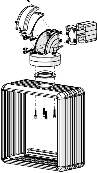
Mounting View Montaj Görünümü
