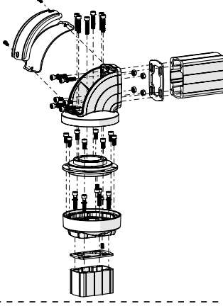
Mounting View Montaj Görünümü
