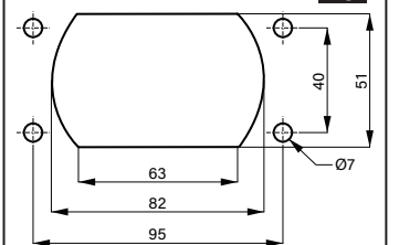
Panel mounting dimensions Pano montaj ölçüleri
