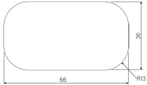
Profile hole dimensions (*) Profil delik ölçüleri (*)
