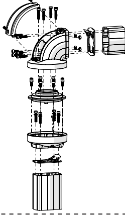
Mounting View Montaj Görünümü
