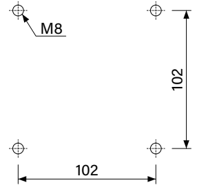
Module mounting dimensions Modül montaj ölçüleri
