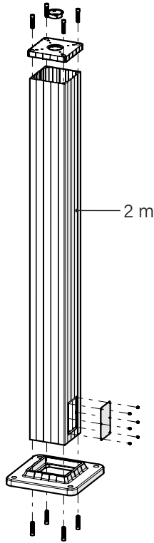
Mounting View Montaj Görünümü
