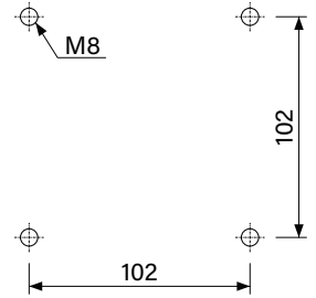
Module mounting dimensions Modül montaj ölçüleri
