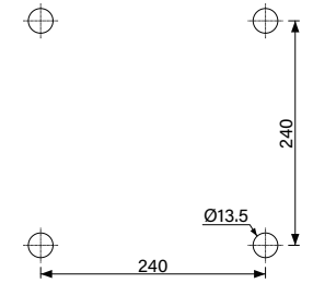
Ground mounting dimensions Zemin montaj ölçüleri
