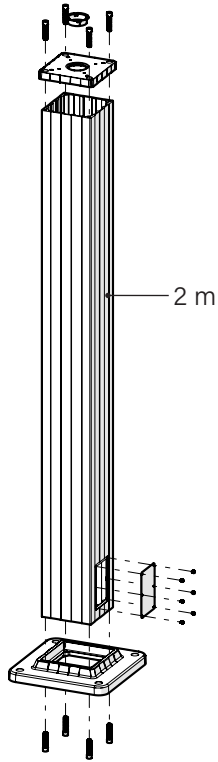
Mounting View Montaj Görünümü
