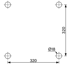
Ground mounting dimensions Zemin montaj ölçüleri
