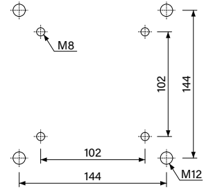
Module mounting dimensions Modül montaj ölçüleri
